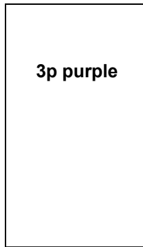
AR5
